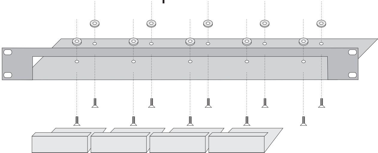
RMK für Singlehead Geräte / RMK for singlehead devices
