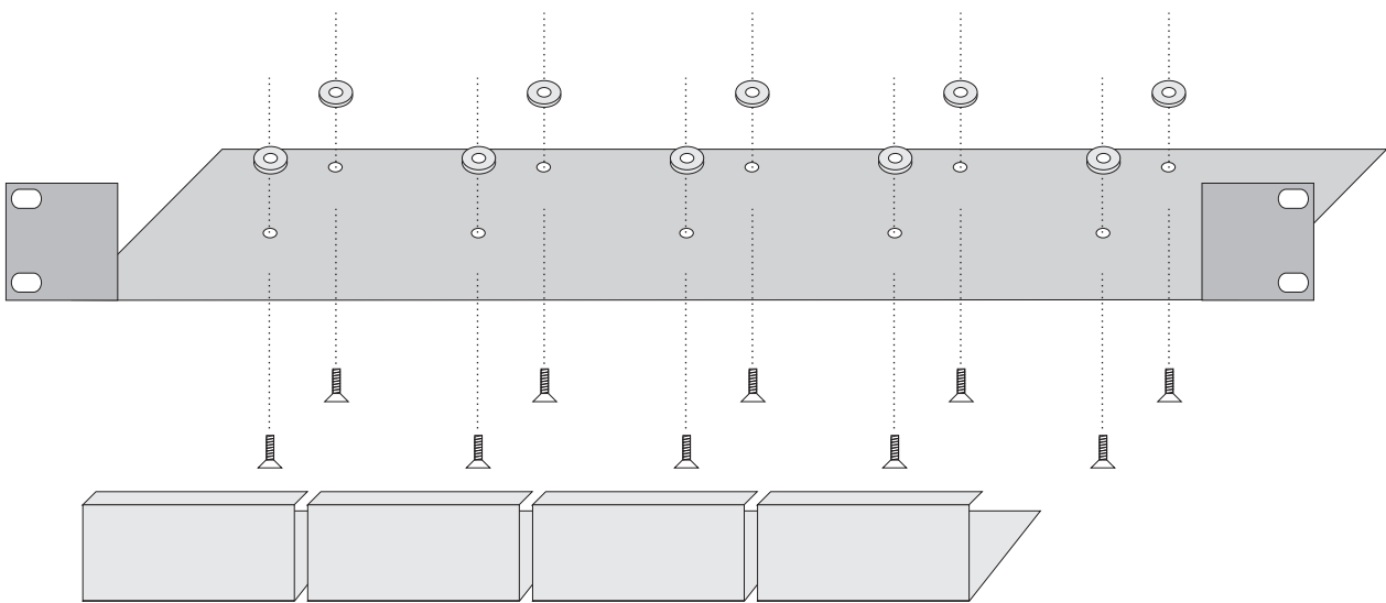
RMK für Dualhead Geräte / RMK for dualhead devices
